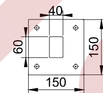
Detalhe A Base Poste esc. 1:10
